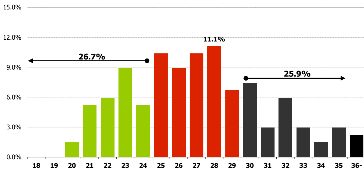
Histogram súčtov kôl
